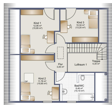
Grundrisskizze 1. OG
